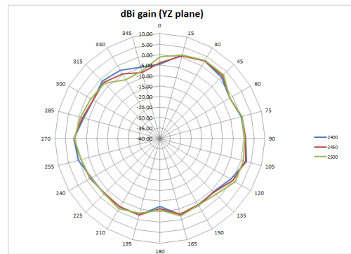
2.4GHz E-Plane
