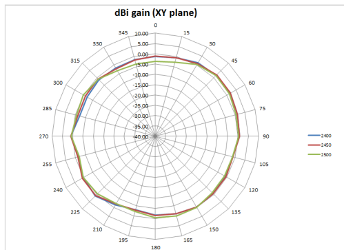
2.4GHz H-Plane
