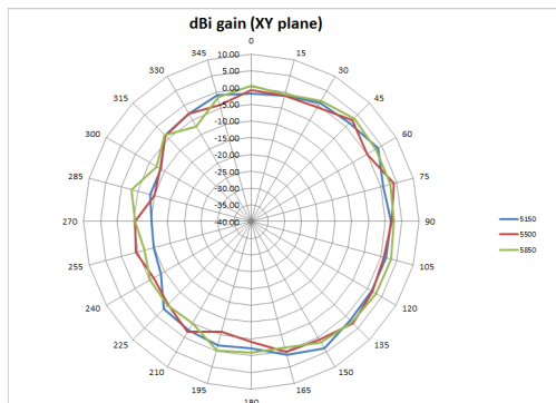
5GHz H-Plane
