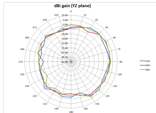
5GHz E-Plane
